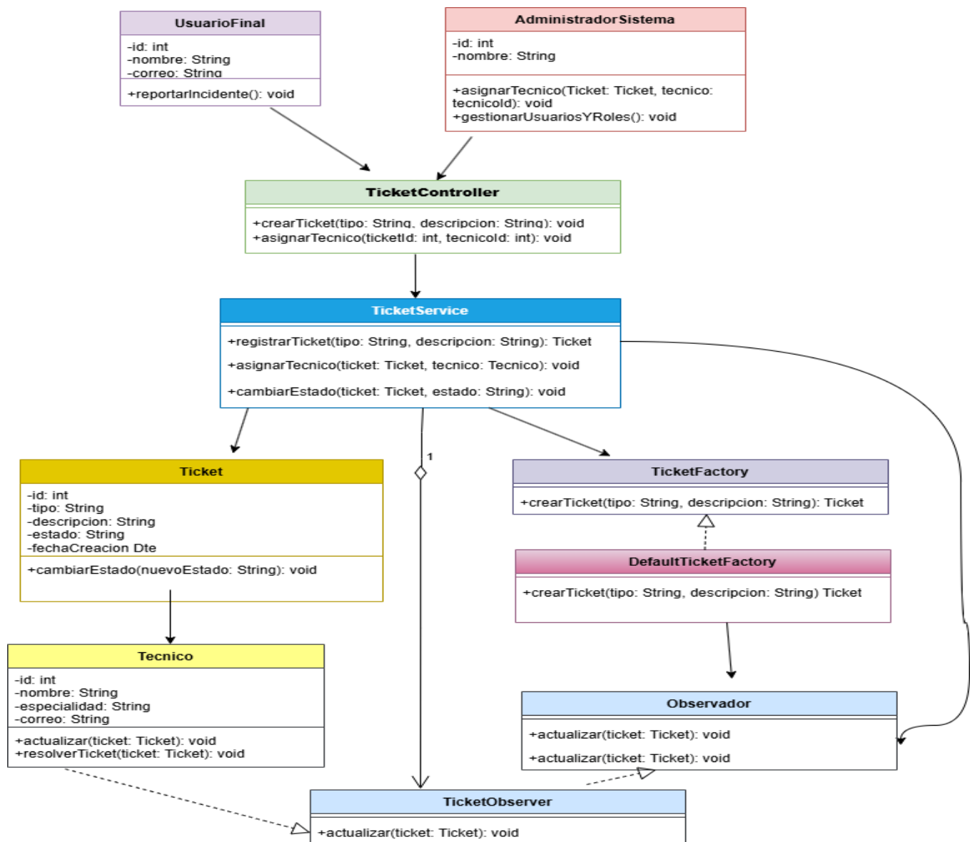
Figura 2. Diagrama de Clases UML.
