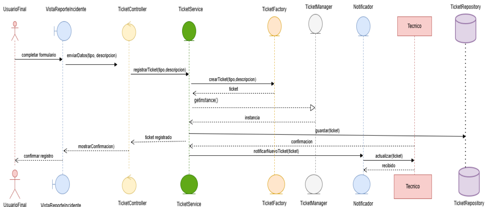
Figura 3. Diagrama de Secuencia.
